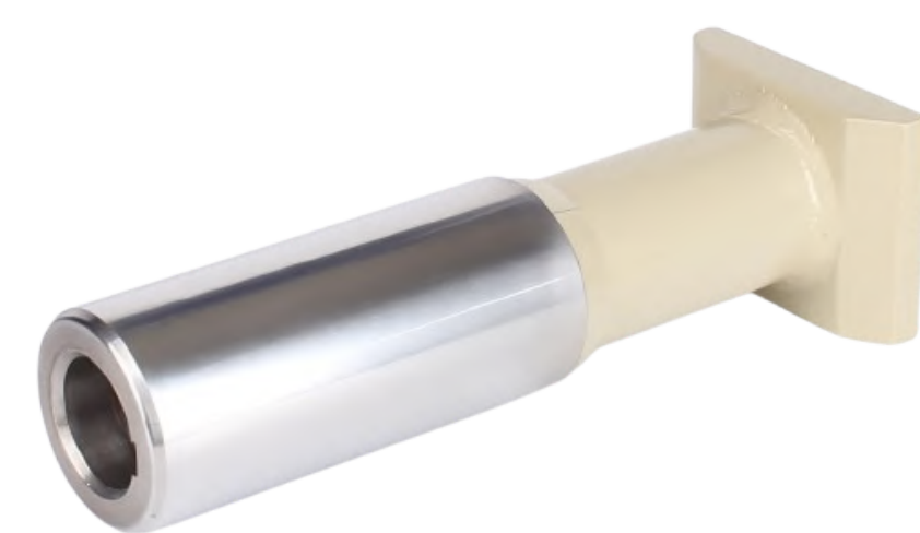
ULM20138 MIXER SHAFT – Ø60 L=250
